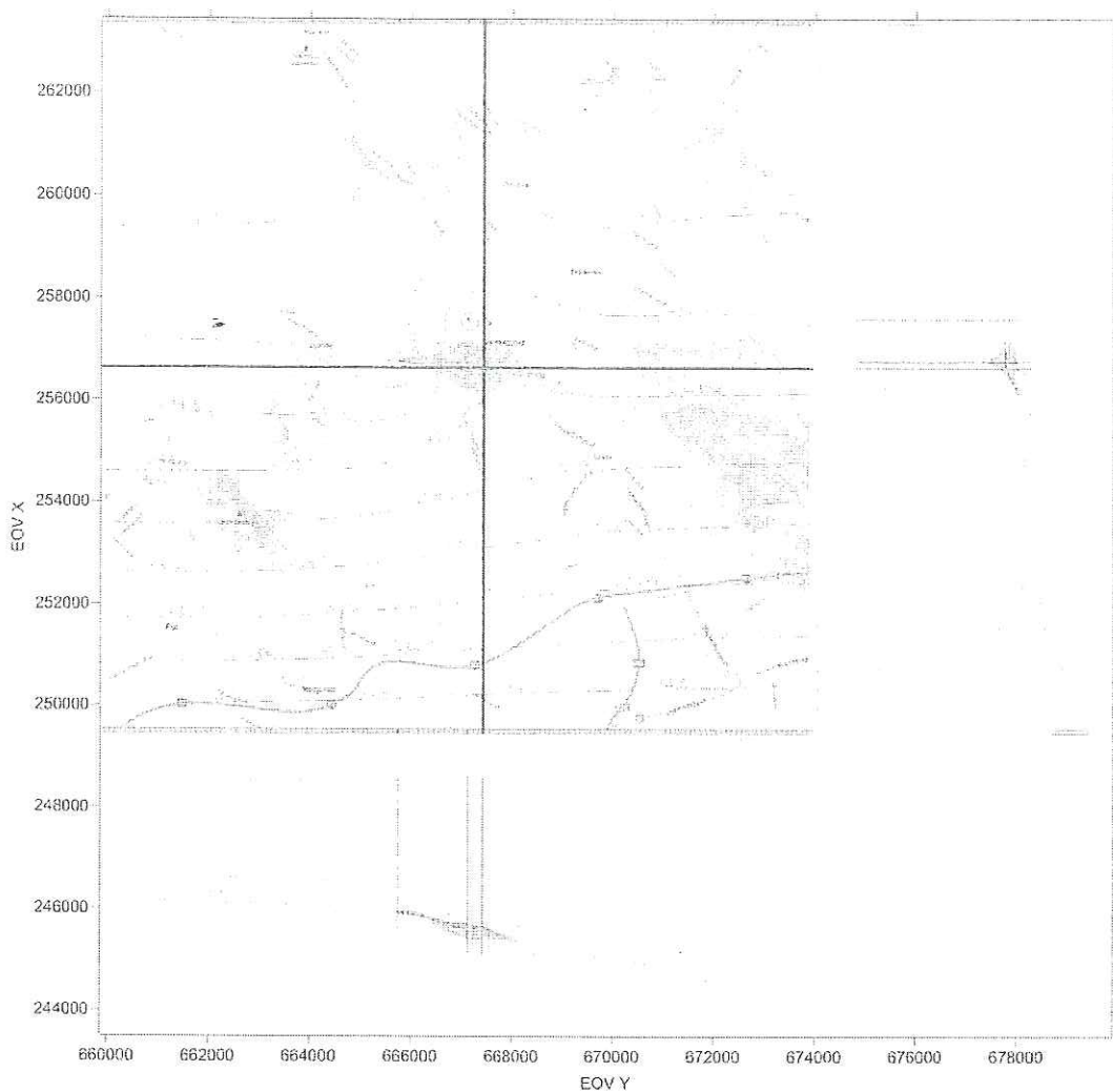
6. ábra A B-15 termelő kutat 6 hónap alatt elérő részecskék pályái (az effektív porozitás értékének tizedrészre való csökkentésével)
