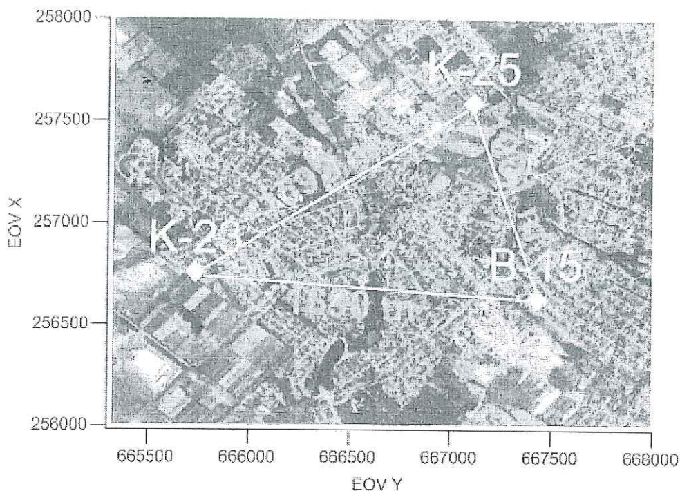
4. ábra: A kutak elhelyezkedése
