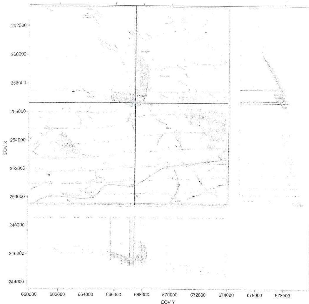
7. ábra A B-15 termelő kutat öt év alatt elért részecskék pályái (az effektív porozitás értékének tizedrészre való csökkentésével)
