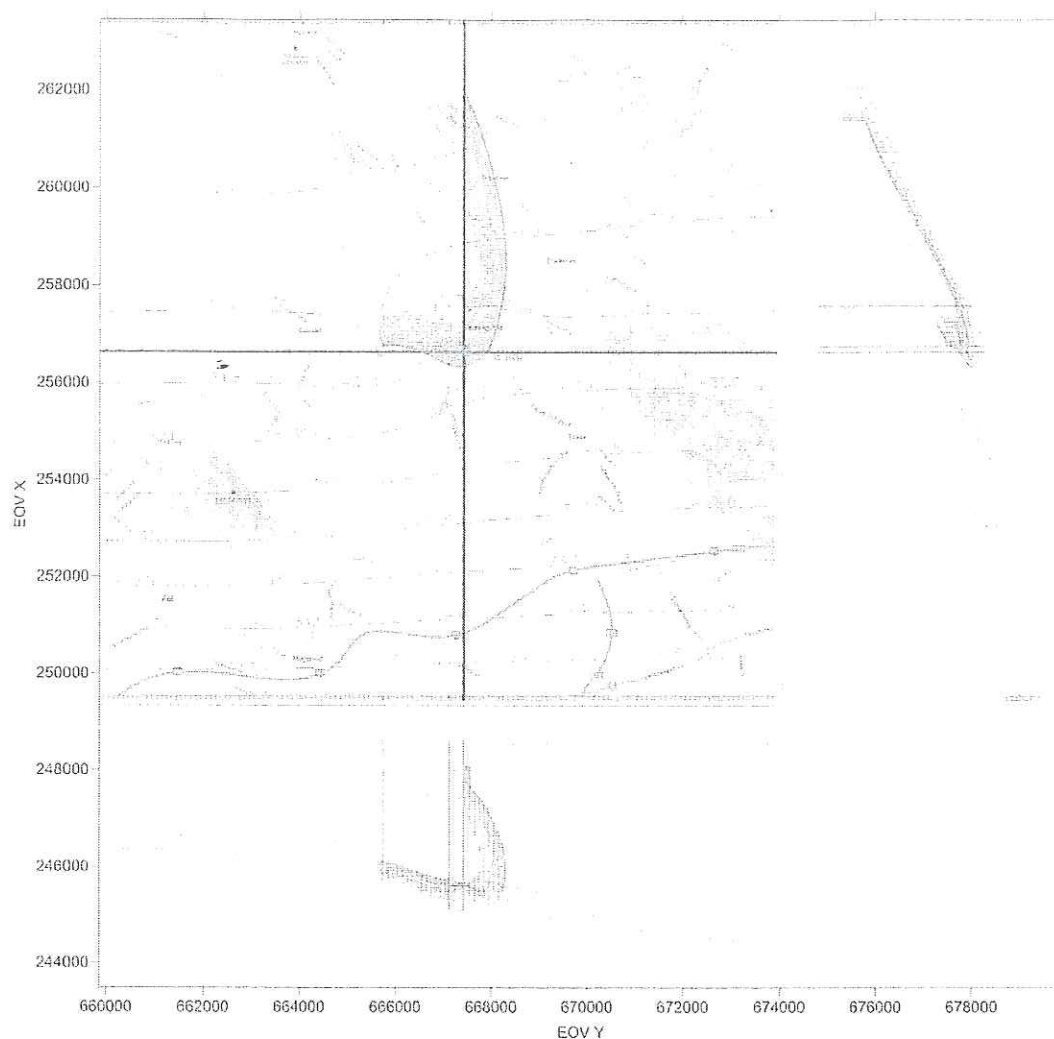
10. ábra A B-15 termelő kutat 50 év alatt elérő részecskék pályái (az effektív porozitás értékének ötödrésze való csökkentésével)
