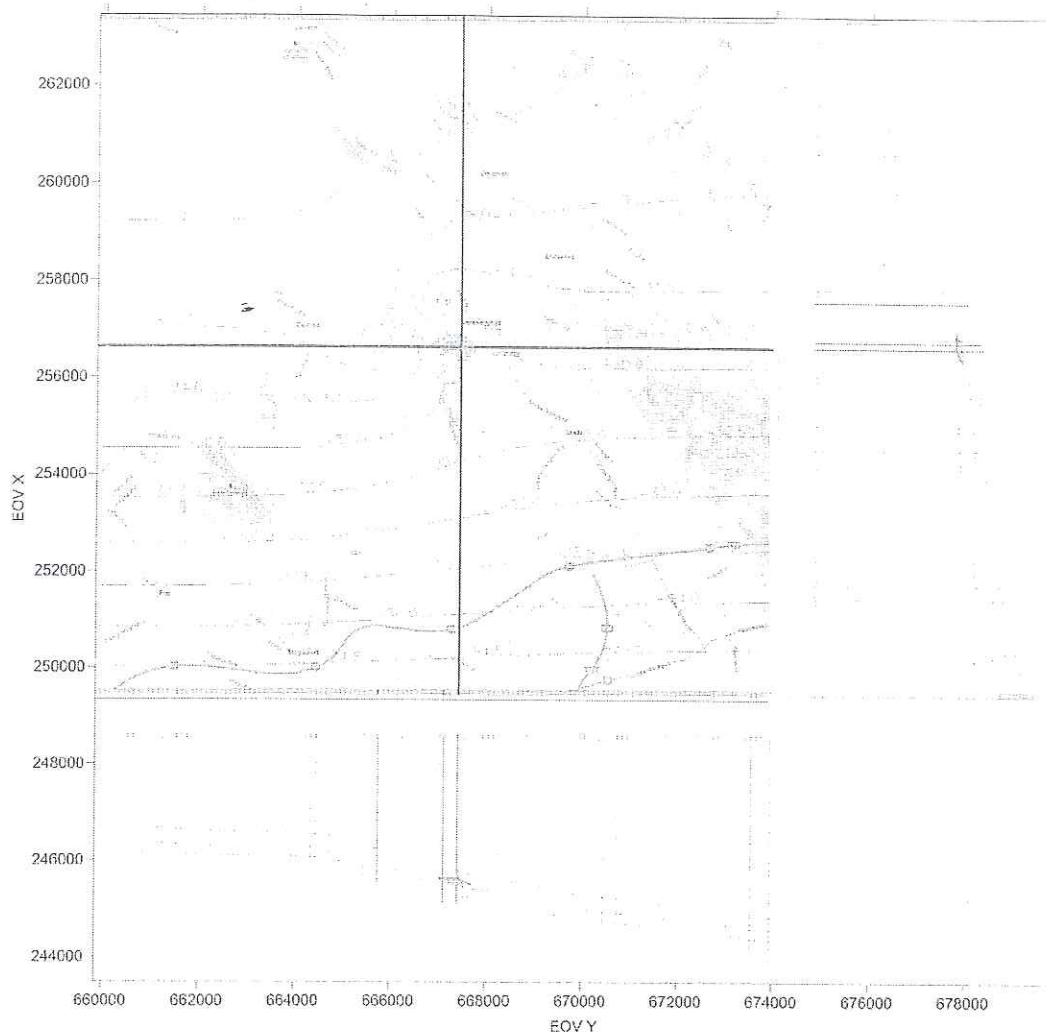
5. ábra A B-15 termelő kutat 20 nap alatt elérő részecskék pályái (az effektív porozitás értékének tizedrészre való csökkentésével)
