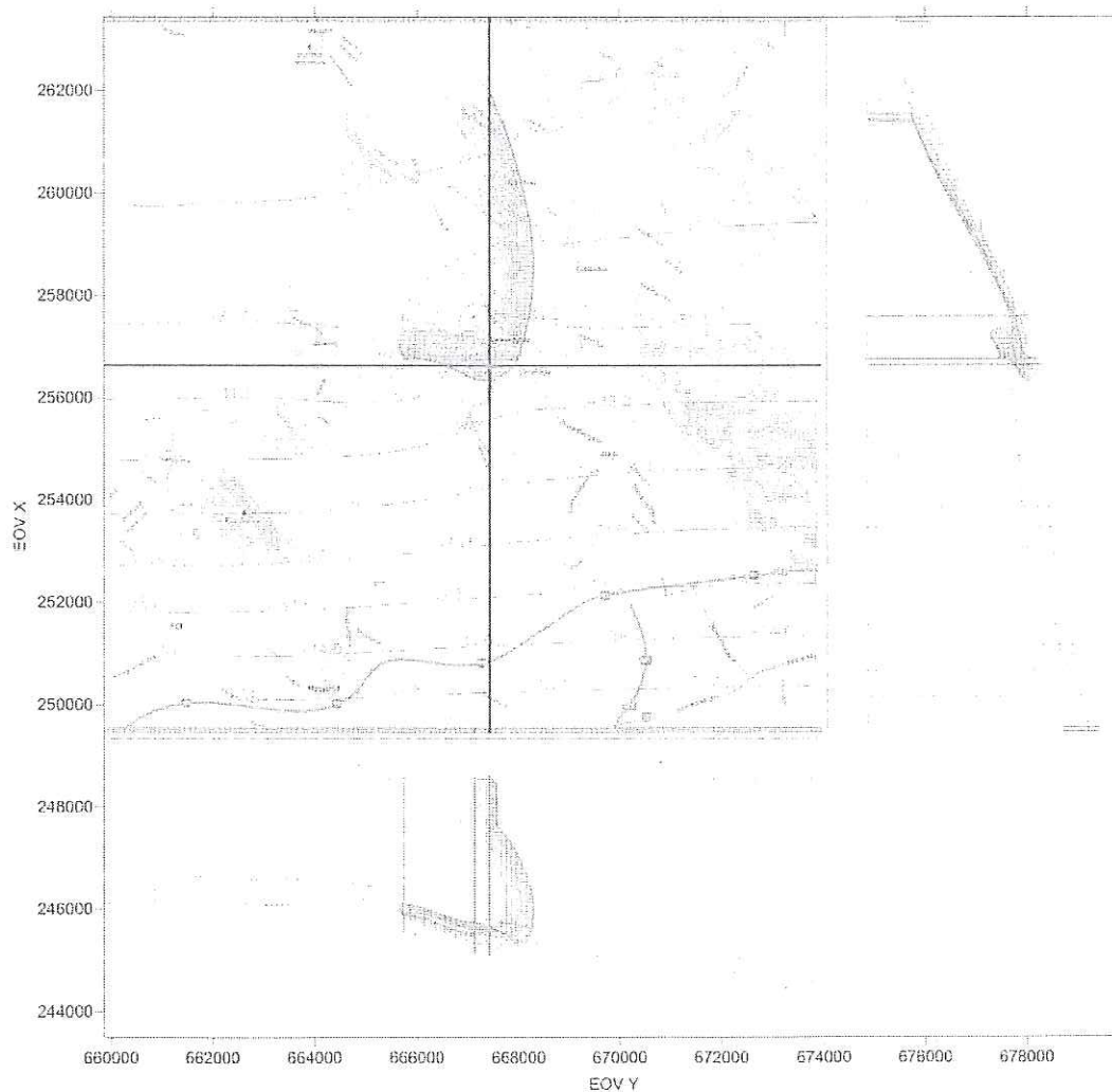
9. ábra A B-15 termelő kutat 50 év alatt elérő részecskék pályái (az effektív porozitás értékének tizedrészre való csökkentésével)
