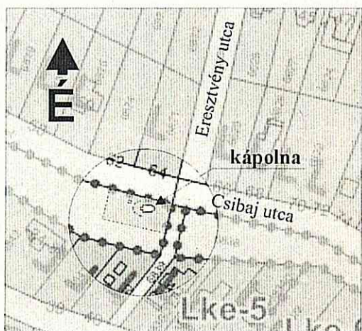
Helyszínrajz
