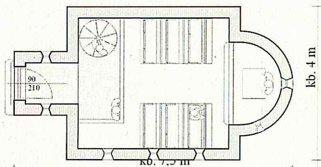
Alaprajz
