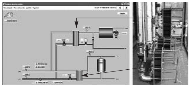
A Misszió Egészségügyi Központ termálvíz ellátását figyelő monitoring rendszer. Az ábrán két hőcserélő látható a és melegvizét (elől) nagyobb a fűtésért (fent) a kisebb (lent) a melegvíz ellátásért felel.
